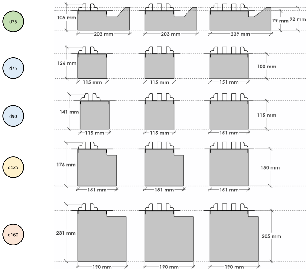
Plenum box + diffuser grill
